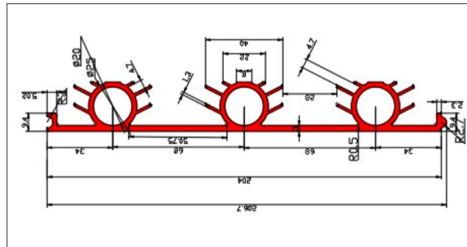
模具号: 8203 壁厚: 2.5mm 米重: 3.6kg/m 蒸发面积: 0.852 m 2
