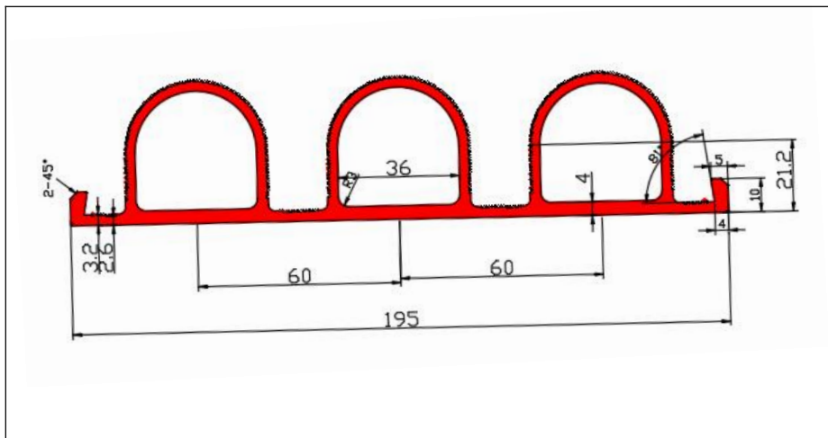
模具号: 8202 壁厚: 3.2mm 米重: 4.5kg/m 蒸发面积: 0.707 m 2
