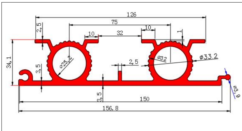
模具号: 6477 壁厚: 3.4mm 米重: 3.74kg/m 蒸发面积: 0.605 m 2
