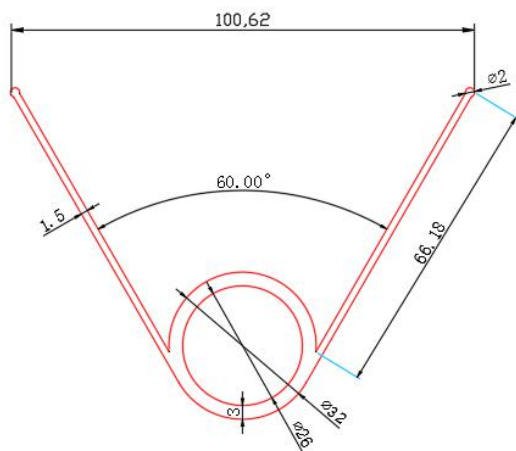
模具号: 8054 壁厚: 3mm 米重: 1.32 kg/m 蒸发面积: 0.369 m 2
