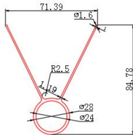
模具号: 7725 壁厚: 2mm 米重: 0.85 kg/m 蒸发面积: 0.345 m 2
