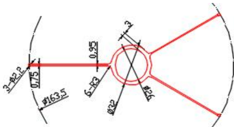
模具号: 6033-3.0 壁厚: 3mm 米重: 1.25kg/m 蒸发面积: 0.491 m 2
