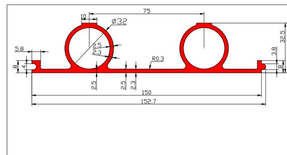
模具号: 8343 壁厚: 2.5mm 米重: 2.3kg/m 蒸发面积: 0.472 m 2
