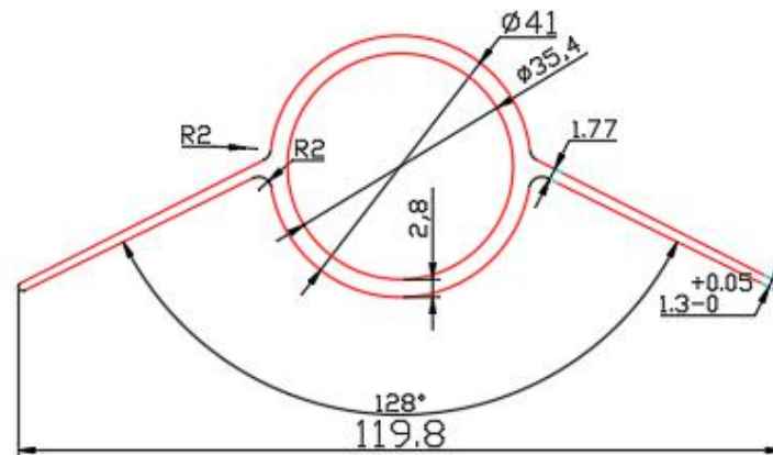
模具号: 8192 壁厚: 2.8mm 米重: 1.4kg/m 蒸发面积: 0.298 m 2
