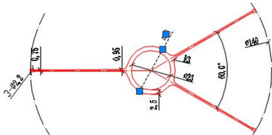
模具号: 7740 壁厚: 2.5mm 米重: 0.98kg/m 蒸发面积: 0.42 m 2
