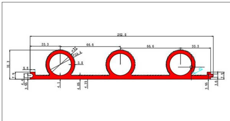
模具号: 8053 壁厚: 2.4mm 米重: 4.62kg/m 蒸发面积: 0.621 m 2
