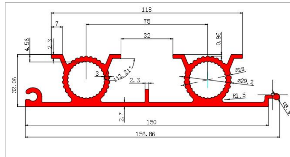
模具号: 8010 壁厚: 3mm 米重: 3.2kg/m 蒸发面积: 0.606 m 2
