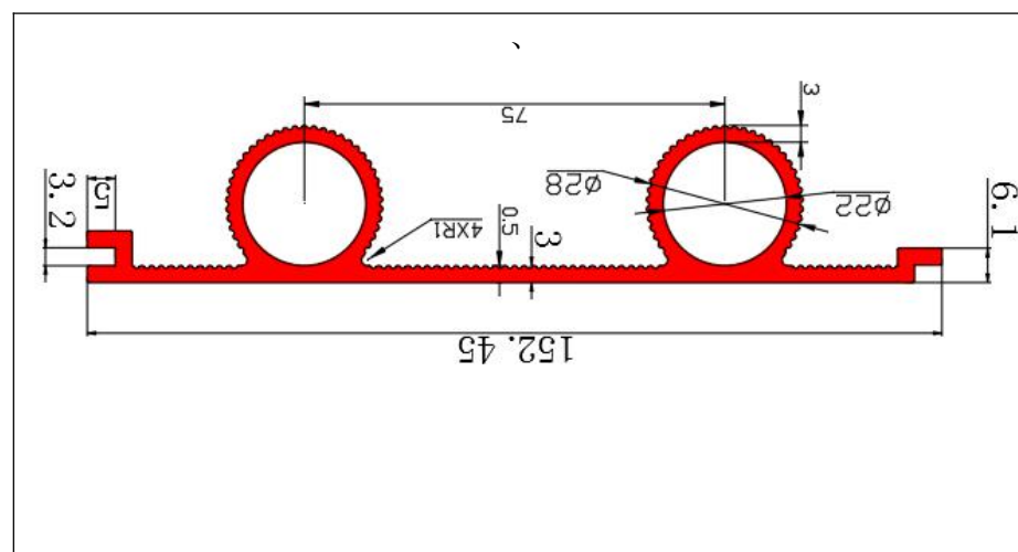
模具号: 7988 壁厚: 3mm 米重: 2.35kg/m 蒸发面积: 0.474 m 2
