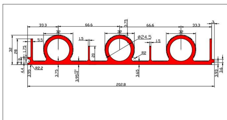
模具号: 8040 壁厚: 3.75mm 米重: 4.79kg/m 蒸发面积: 0.771 m 2
